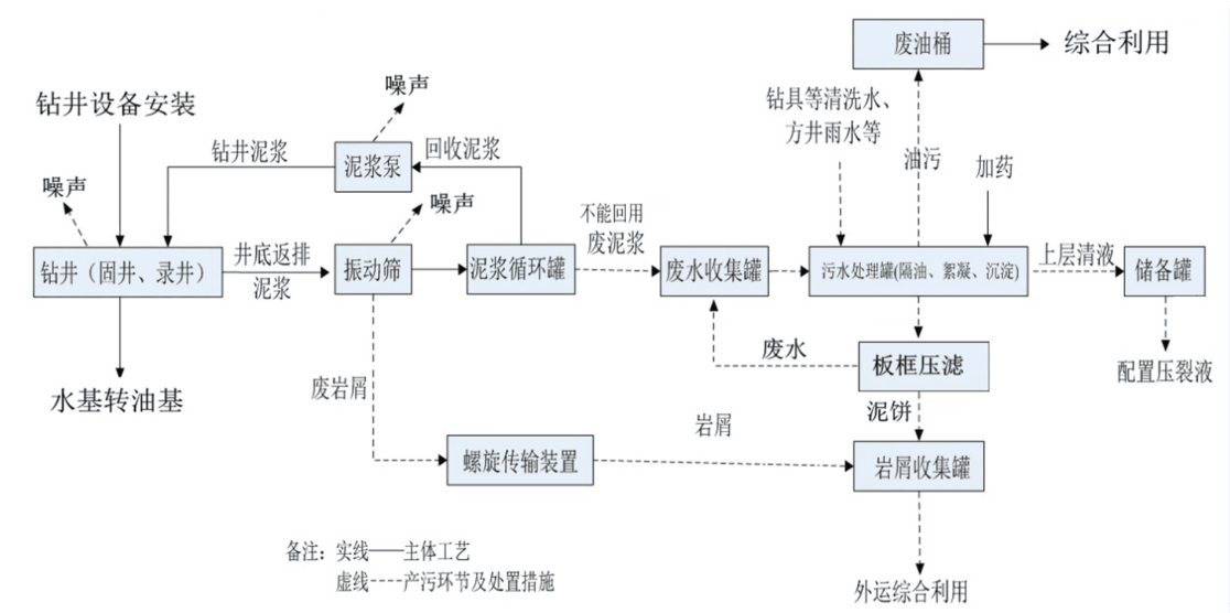
图 2.4-2 钻井工艺流程及产排污环节图
