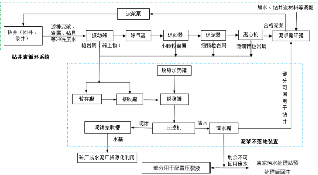
图 2.4-3 项目钻井液循环系统工艺流程图
